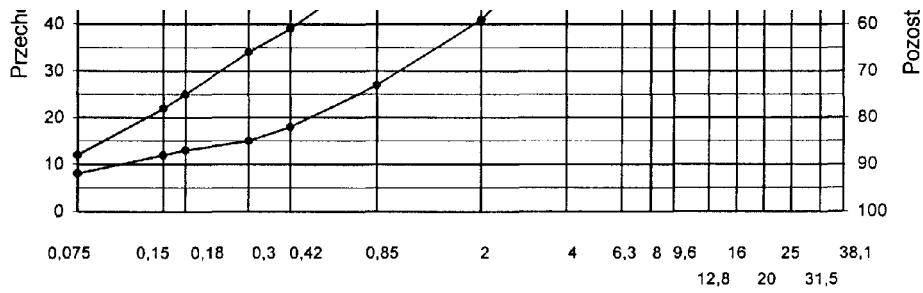
Wymiary oczek sit kwadratowych, mm
