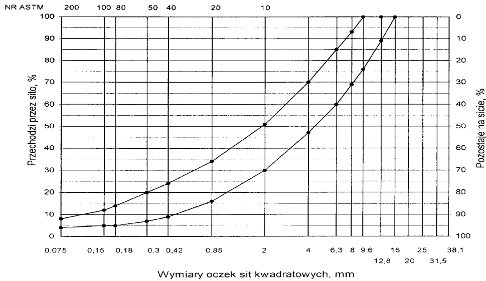
Rys. 5. Krzywe graniczne uziarnienia mieszanki mineralnej BA od 0 do 12,8 mm do podbudowy nawierzchni drogi o obciążeniu ruchem KR 1 lub KR 2
