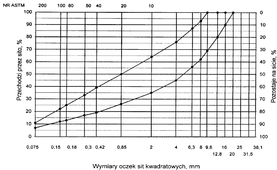
graniczne uziarnienia mieszanki mineralnej BA od 0 do 16mm, od 0 do 12,8 mm do warstwy ścieralnej nawierzchni drogi o obciążeniu ruchem KR1 lub KR2
