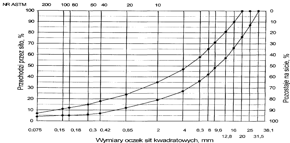
Rys. 7. Krzywe graniczne uziarnienia mieszanki mineralnej BA od 0 do 25 mm podbudowy
