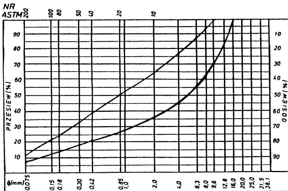
Rys. 1. Krzywe graniczne uziarnienia mieszanki mineralnej 0÷20 mm do warstwy ścieralnej z betonu
