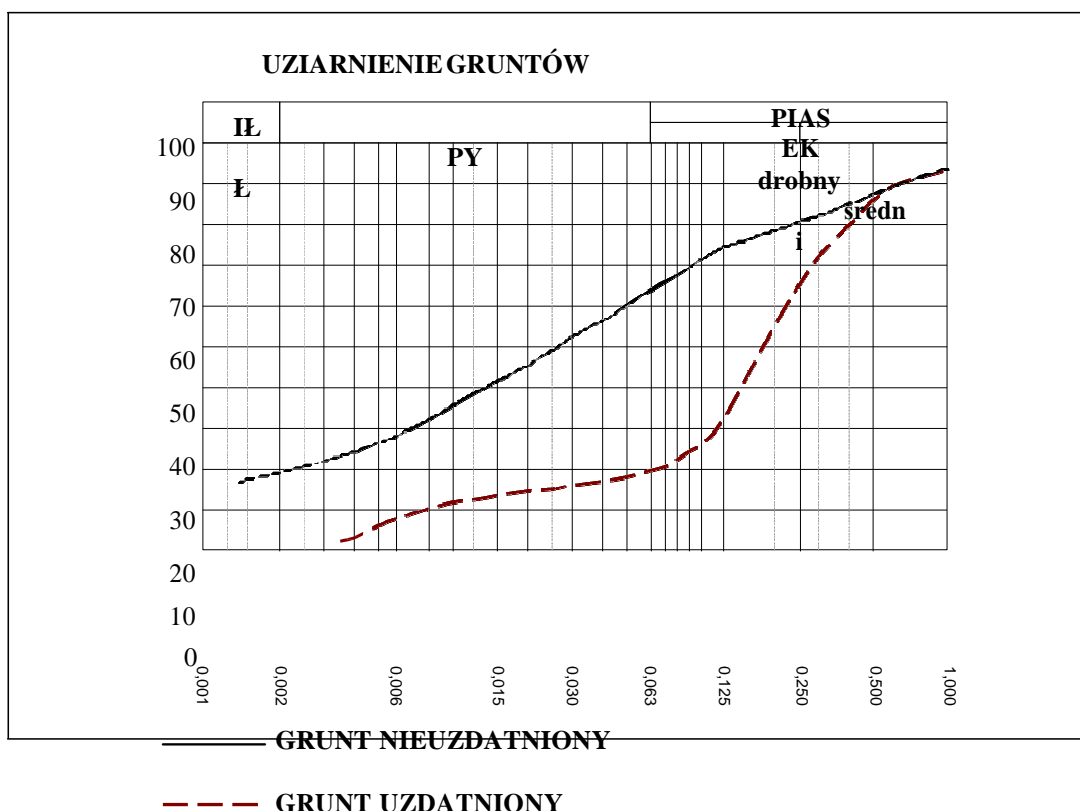
Rysunek 1 - Optymalne uziarnienie wstępne
